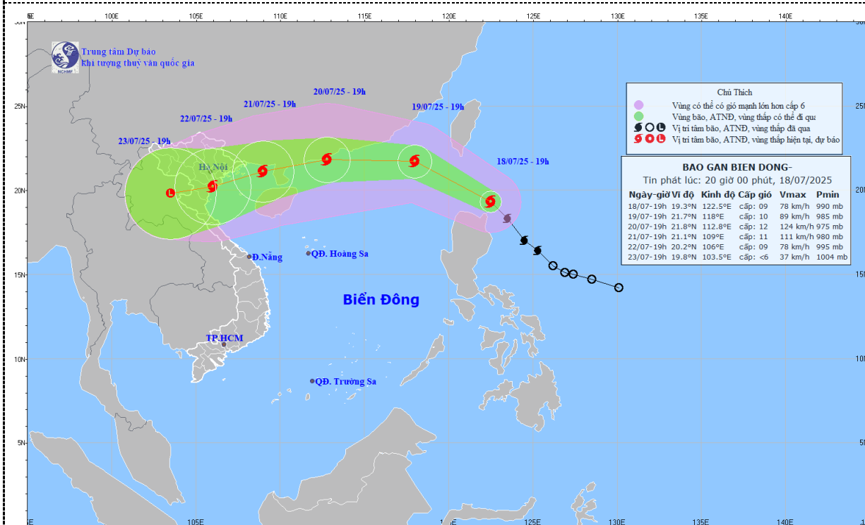
Hình1. Bản đồ dự báo quỹ đạo và cường độ bão Wipha phát lúc 20h00 ngày 18/7/2025
